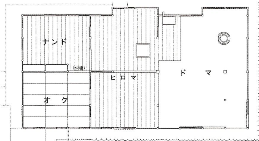
図1 主屋 平面図
